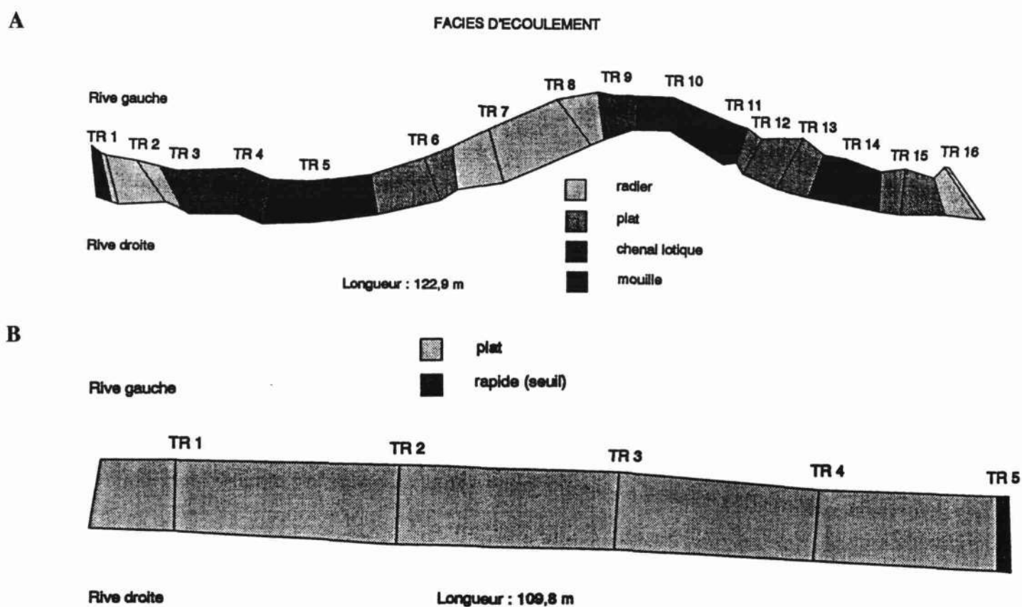
Figure 4.10 : Cartographie des faciès d'écoulement sur la station de référence (A) et la station aménagée (B) de l'Eau Morte.
