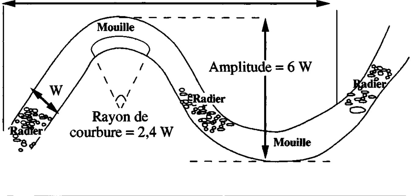
Figure 2.4 : Relations entre la géométrie du lit et la largeur au débit de plein bord ( W ).
