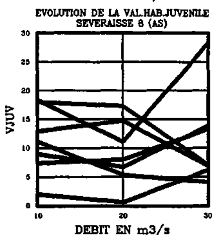
Figure 7.10 : La Severaisse (Hautes Alpes) : Profils d'évolution des vitesses médianes (VI50) et des valeurs d'habitat pour les adultes et juvéniles de truite fario en fonction du débit sur une station de référence (St. 8, AS) et sur une station chenalisée (St1, GS). D'après MALAVOI, 1990.
